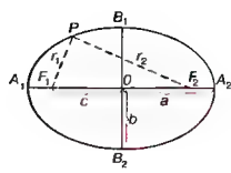
Еліпіс Точки F 1 та F 2 – фокуси еліпса, O – центр еліпса, відрізки: A 1 A 2 – велика вісь еліпса, B 1 B 2 – мала вісь еліпса
